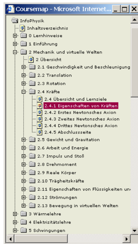
Bild 12: Navigationshilfe ‚Coursemap‘
